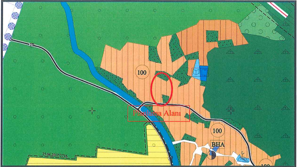
Yürürlükteki Osmangazi Belediyesi Nazım İmar Planı Örneği
