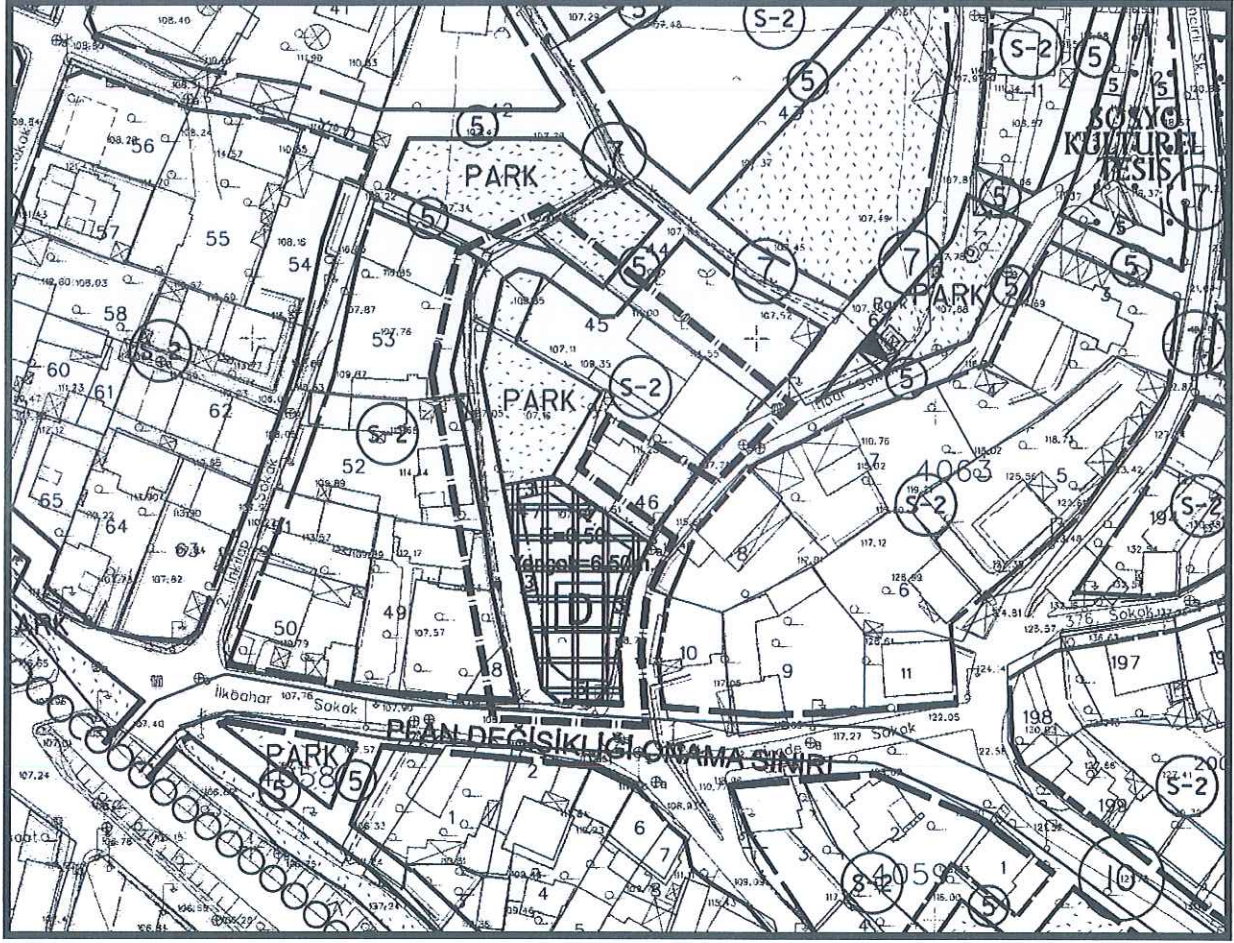
Öneri 1/1000 Ölçekli İsmetiyeköy Mahallesi Uygulama İmar Planı Revizyonu Plan Değişikliği
