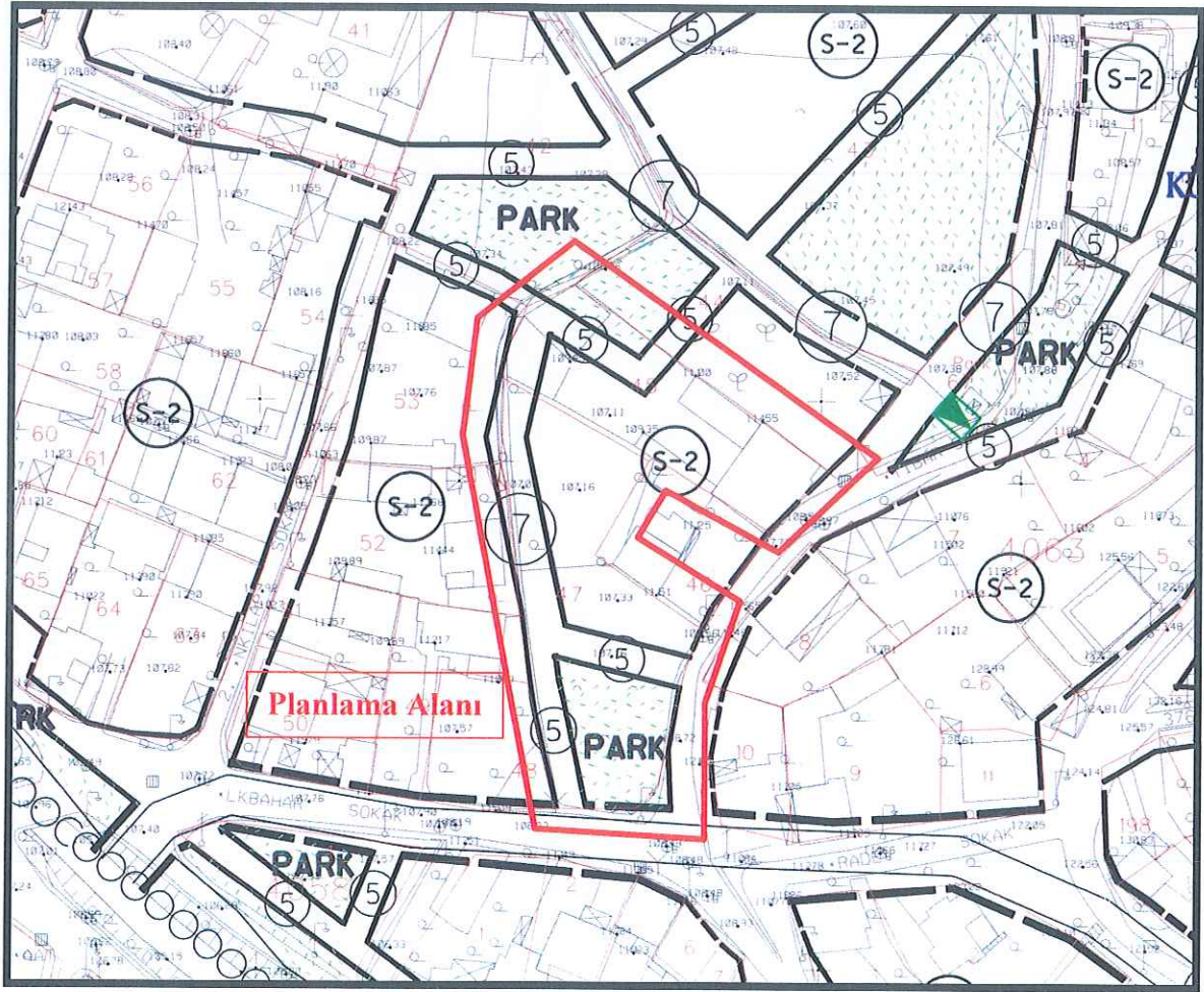
Yürürlükteki 1/1000 Ölçekli İsmetiyeköy Mahallesi Uygulama İmar Planı Revizyonu
