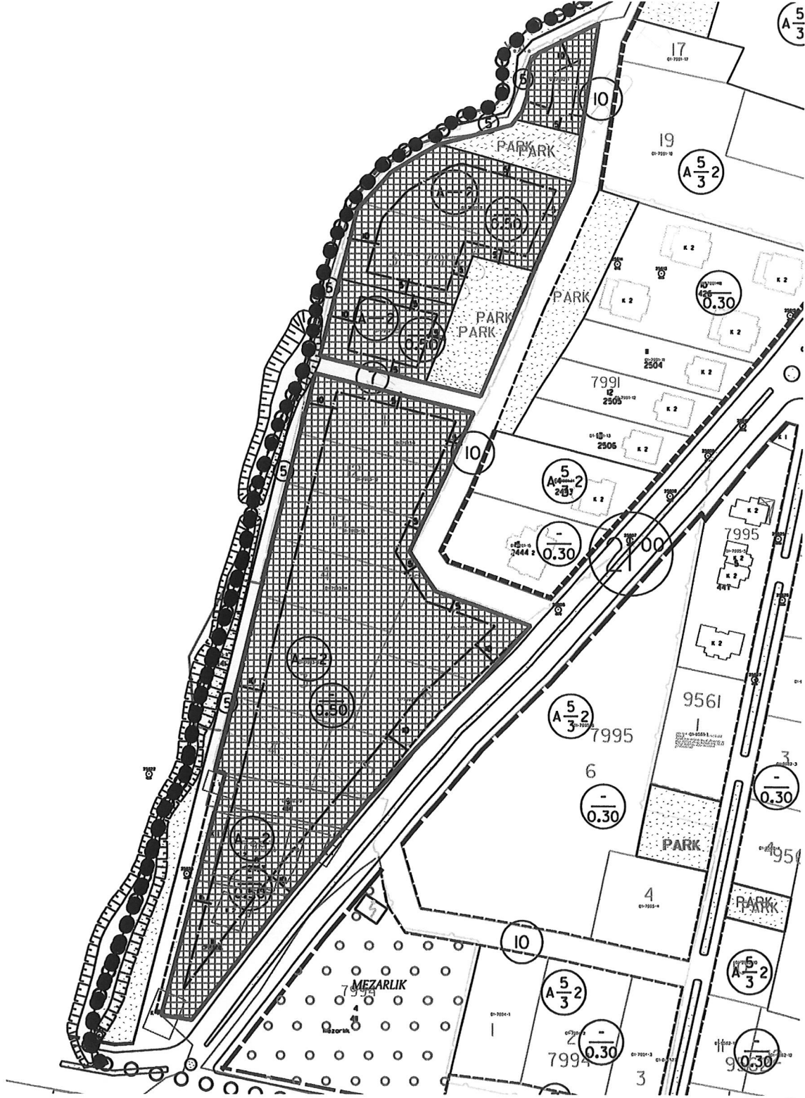
Şekil 9. Onaylı 1/1000 ölçekli Yalova Yolu UİP örneği
