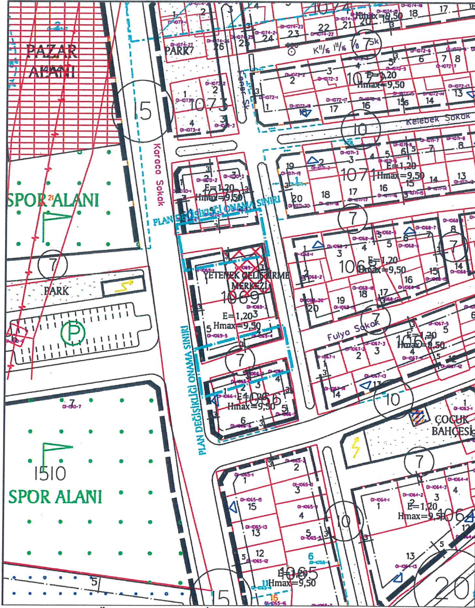
Resim 3: 1/1000 Ölçekli Uygulama İmar Planı Değişikliği
